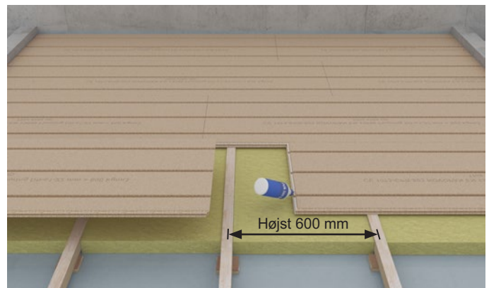
Figur 5 Klimagulv lagt i forbandt med flyvestød og pladeforskydning på mindst 300 mm. Må kun anvendes i almindelige boligrum.
